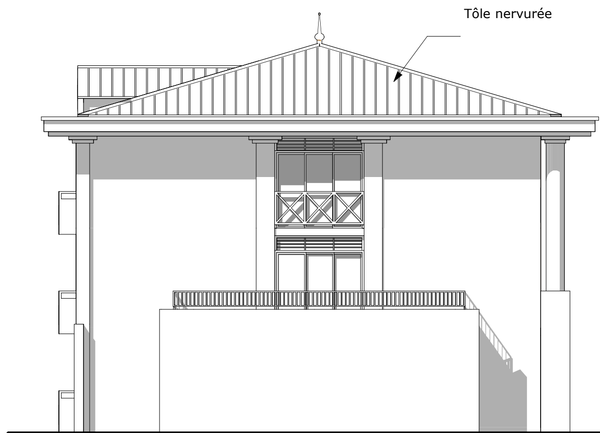
Elévation Sud sur pignon
