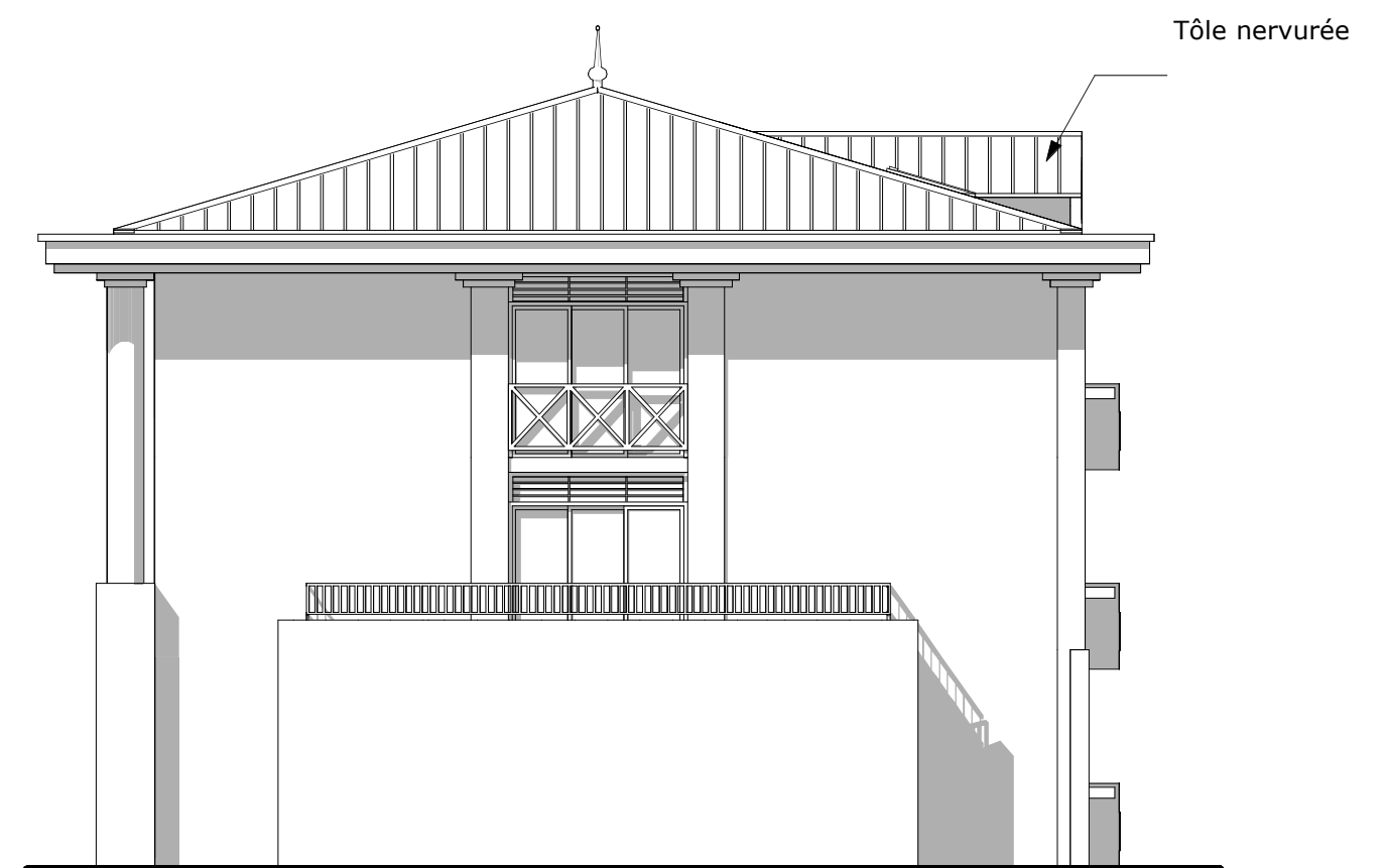
Elévation Nord sur pignon
