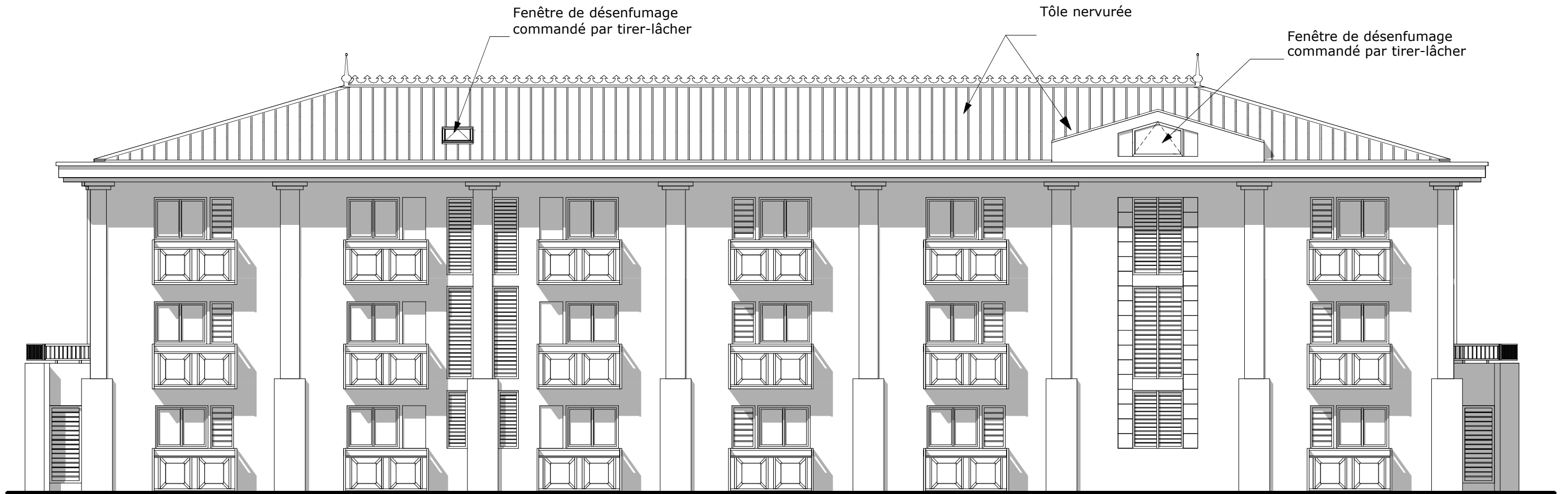
Élévation Ouest sur chambres
