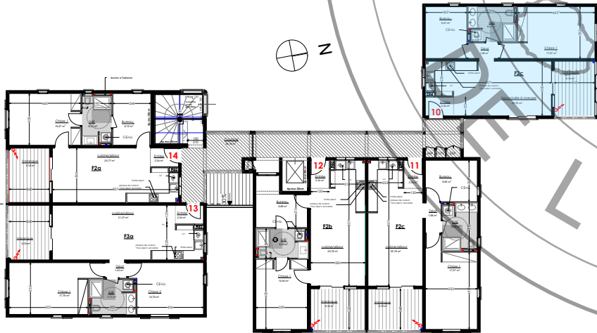
niveau R+1
